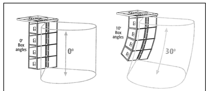
Abb.3: Beispiel für ein segmentiertes Line Array mit 0°(links) und 30°(rechts) Öffnungswinkel
