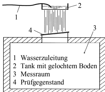
Abbildung 1: Messprinzip zur Erfassung von Regengeräuschen im Prüfstand.
