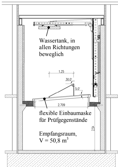
Abbildung 2: Aufbau des Regengeräuschprüfstands im IBP.
