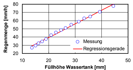
Abbildung 4: Regenmenge in Abhängigkeit von der Füllhöhe des Wassertanks. Die Messungen wurden an einem Tank für starken Regen (Lochdurchmesser 1,0 mm) durchgeführt.
