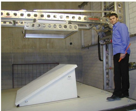
Abbildung 3: Wassertank (aus transparentem Kunststoff) mit Positioniereinrichtung über der Einbaumaske für kleine Bauelemente.
