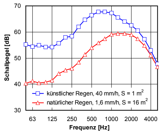
Abbildung 5: Frequenzspektren von natürlichem und künstlichem Regen. Die Messungen erfolgten an einer Dachkonstruktion aus ETFE-Folienkissen.
