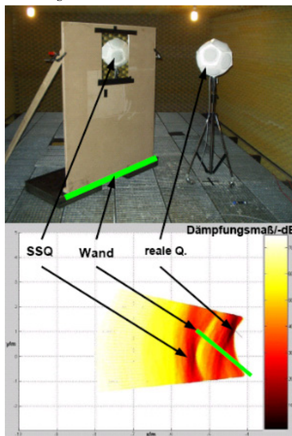
Abbildung 2: Das obere Bild zeigt einen Messaufbau im reflexionsarmen Raum. Die Reflexion, die das Schallfeld an der Wand erfährt, kann durch die SSQ (Spiegelbild) beschrieben werden. Im unteren Bild ist das Ergebnis der überlagerten RIR zu sehen. Die Direktschallquelle (reale Q.) und die SSQ werden durch je ein Maximum repräsentiert.
