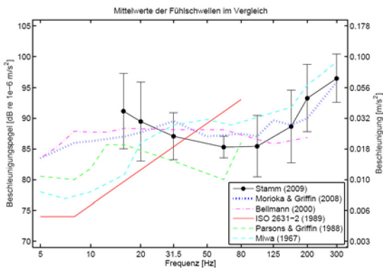
Abbildung 4: Fühlschwellen für Sinussignale (Ganzkörperschwingungen).
