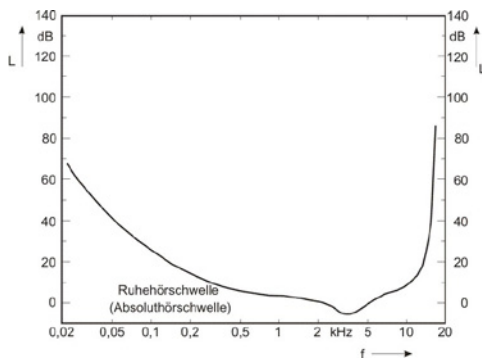
Abbildung 3: Hörschwelle (nach Stevens 1975).
