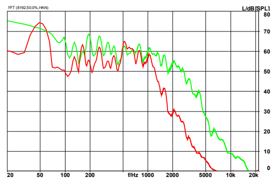
Abbildung 2: Korrelation zwischen akustischem und vibratorischem Signal am Sitz (FFT-Analyse, FFT-Länge 8192).
