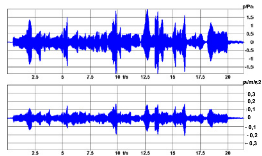
Abbildung 1: oben: zeitliche Sequenz einer Luftschallaufnahme von einem Orgelstück; unten: zeitliche Sequenz der Schwingungsaufnahme.
