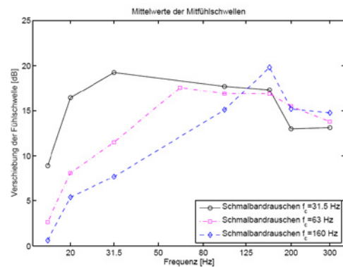
Abbildung 5: Mittelwerte der Mitfühlschwellen für Sinussignale unterschiedlicher Frequenzen bei Maskierung durch ein Schmalbandrauschen mit f_c=31.5 Hz, 63 Hz und 160 Hz.
