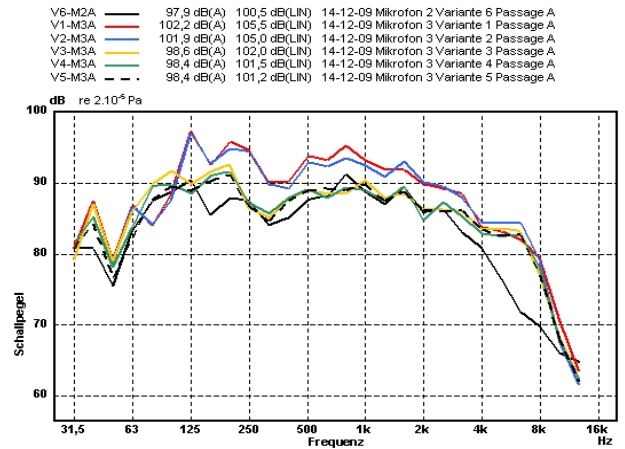
Abbildung 3: Messergebnis L_{Aeq} A vor Trompeten [dB(A)]
