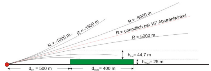
Abb. 1 Veranschaulichung der Aufteilung der Schallbeiträge bei Anwesenheit eines Waldstückes im Ausbreitungspfad
