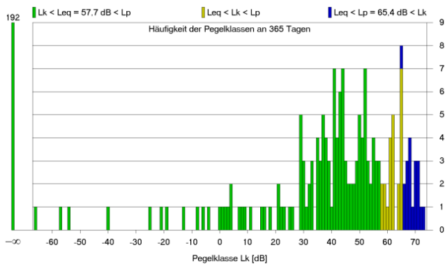
Abb. 1 Häufigkeitsverteilung des Tagesmittelungspegels in einem Ort nahe eines Schießplatzes (klassiert in 1-dB-Klassen).
