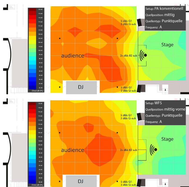
Abbildung 1: Verteilung des A-bewerteten Schallpegels im Club für eine mittig angeordnete Schallquelle bei Links-Rechts-Beschallung (oben) bzw. bei WFS (unten)
