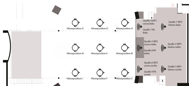
Abbildung 2: Aufteilung Hör- und Quellpositionen im Hörversuch Ortung
