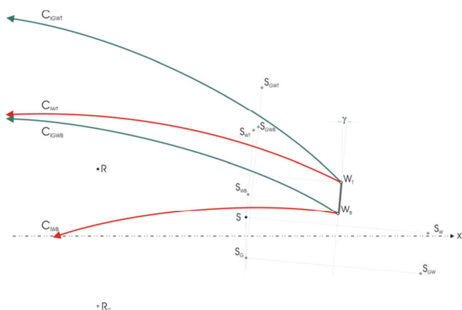
Abbildung 2 Skizze zur Reflexionsbedingung für den Fall „Inversion“ (x markiert die Bodenebene, alle übrigen Bezeichnungen nach Tabelle 1)
