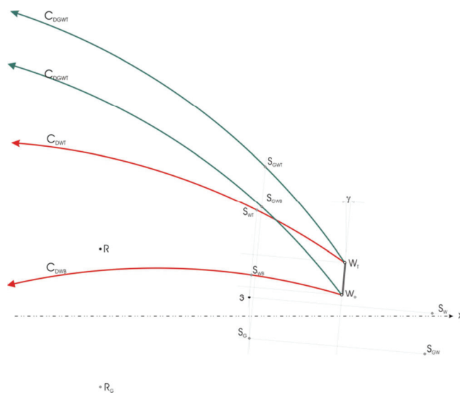
Abbildung 1 Skizze zur Neigungsbedingung für den Fall „Mitwind“ (x markiert die Bodenebene, alle übrigen Bezeichnungen nach Tabelle 1)
