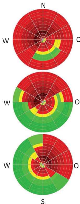
Abb. 2 Quellbezogene Lärmrosen für die Profilprognosen nach Abb. 1 (oben: 07 bis 08 Uhr, Mitte 08 bis 09 Uhr, unten: 09 Uhr bis 10 Uhr)
