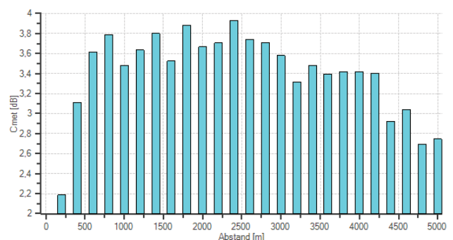
Abb. 3 Abstandsabhängigkeit des C met für die Wintermonate 12.2013 bis 02.2014 für die Schallausbreitungsrichtung West
