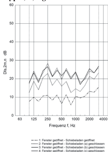
Abbildung 3: Schallpegeldifferenz, Fenster geöffnet
