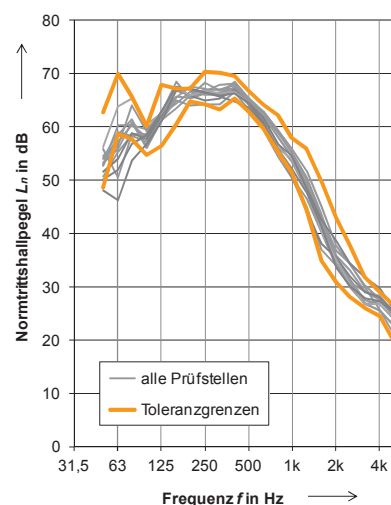
Bild 2: Prüfstellenergebnisse der Trittschallmessung mit berechneten Toleranzgrenzen
