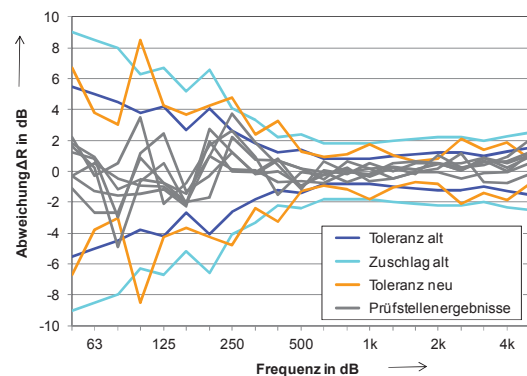
Bild 1: Abweichungen der Luftschallergebnisse der Prüfstellen vom Vergleichswert mit bisherigen und neuen Toleranzgrenzen
