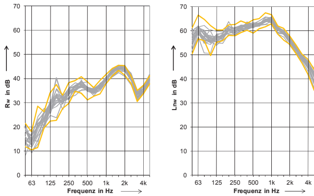
Bild 3: Messergebnisse der VMPA-Prüfstellen für Luft- und Trittschall
