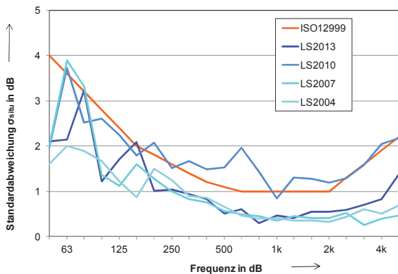
Bild 4: Standardabweichungen der Luftschallmessungen im Vergleich mit den Unsicherheiten der DIN EN ISO 12999
