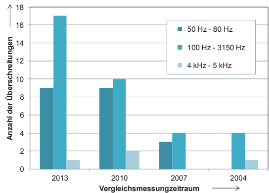
Bild 9: Verteilung der Überschreitungen, Luftschaall
