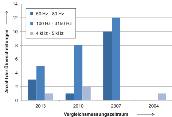
Bild 10: Verteilung der Überschreitungen, Trittschaall
