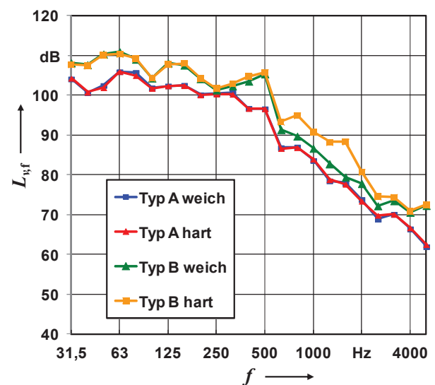
Bild 4: Freie Schnelle in dB re 5e-8 m/s, modifizierte Hammerwerke Typ A und Typ B hart und weich gelagert an den Füßen
