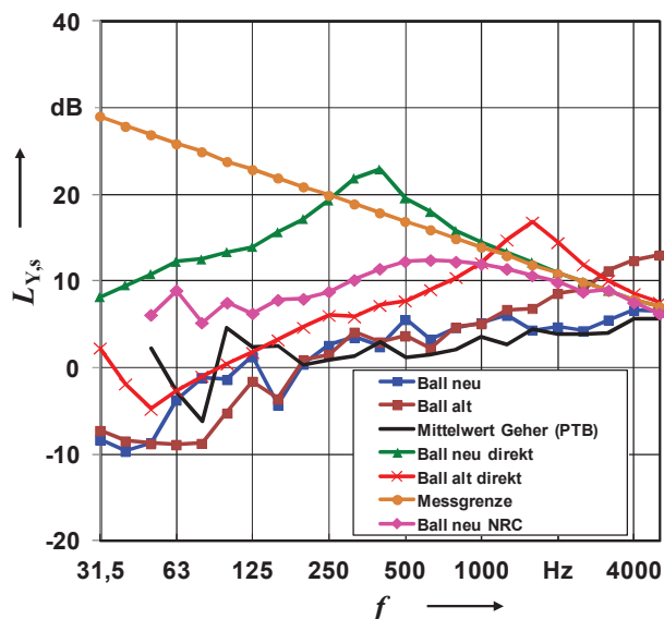
Bild 11: Vergleich der Mobilität der Gummibälle in dB re 2,5e-3 m/N/s, direkte Messung und 2-Platten-Verfahren
