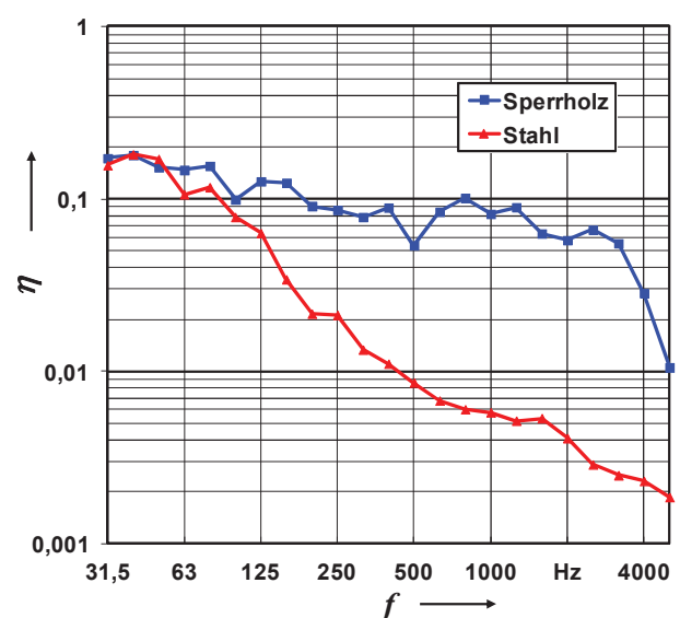
Bild 1: Verlustfaktoren der verwendeten Empfangsplatten
