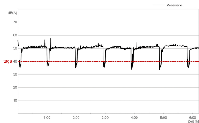
Abbildung 1: Pegel-Zeit-Verlauf, Messung am Immissionsort Freisitz in ca. 4 m Abstand zur Luft/Wasser-Wärmepumpe, rot-gestrichelt: um 10 dB reduzierter Immissionsrichtwert tags für ein reines Wohngebiet.
