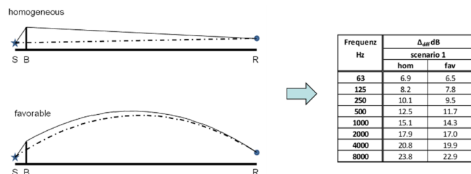
Abbildung 5: Eine 10 m hohe Lärmschutzwand in 50 m Abstand von der Quelle S -> berechnete Pegelminderung ca. 15 dB
