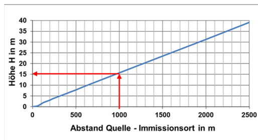
Abbildung 4: Die Höhe des gekrümmten Strahls im Scheitelpunkt
