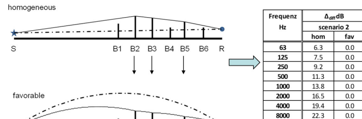
Abbildung 6: Szenario 2 mit mehreren Schirmen B1 bis B6
