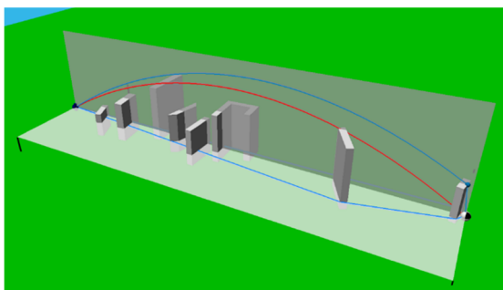
Abbildung 13: Objektanordnung einer Testaufgabe aus ISO/DTR 17534-4
