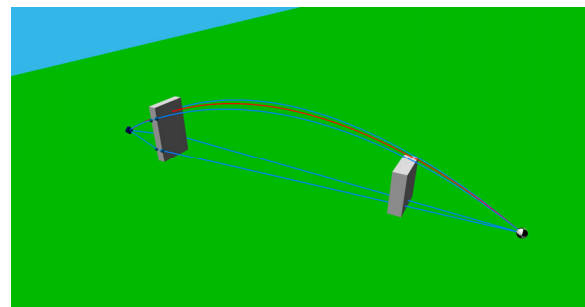
Abbildung 12: Die zur Beugungsrechnung verwendeten unteren Strahlen scheinen das rechte Hindernis zu durchdringen – sie sind aber nur die Projektion des durch das zweite Hindernis nicht blockierten in der Vertikalen gekrümmten Strahlwegs
