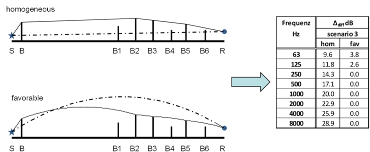
Abbildung 7: Szenario 3 mit Schirm B aus Szenario 1 und den Schirmen B1 – B6 aus Szenario 2
