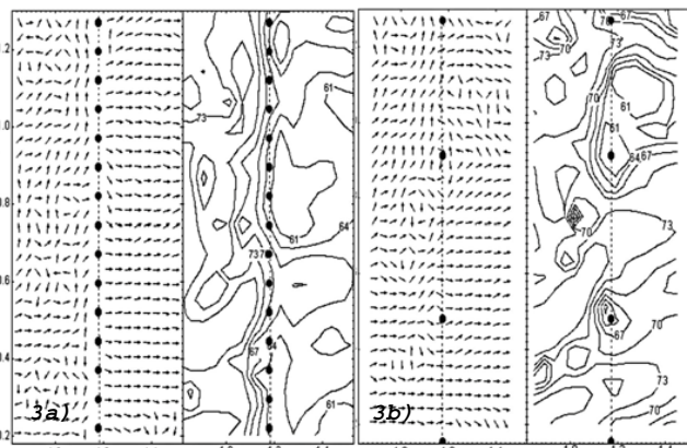
Abb. 3: Intensität (links: Richtung, rechts: Betrag [dB]) auf der Platte bei Anregung auf der linken Plattenseite (a) Rippe mit 16 Schrauben, b) Rippe mit 4 Schrauben an Platte befestigt
