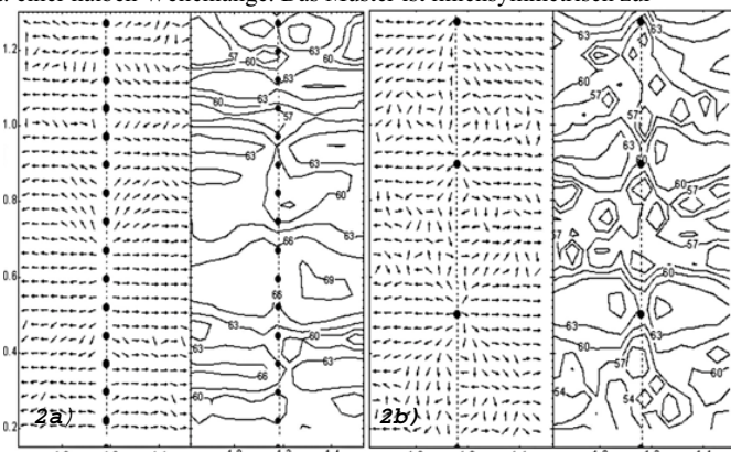
Abb. 2: Intensität (links: Richtung, rechts: Betrag [dB]) auf der Platte bei Anregung der Rippe (a) Rippe mit 16 Schrauben, b) Rippe mit 4 Schrauben an Platte befestigt
