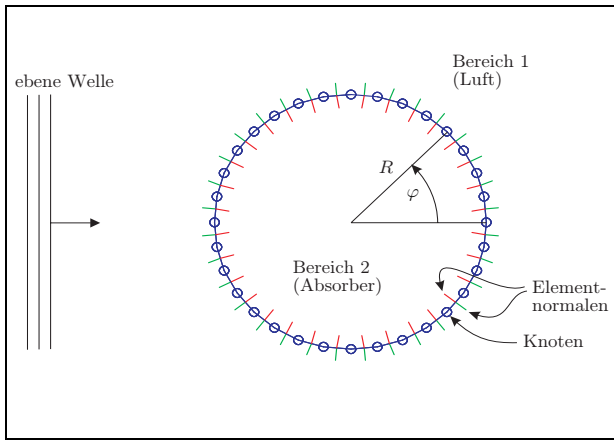
BILD 1. Einfall einer ebenen Welle auf einen Absorberzylinder
