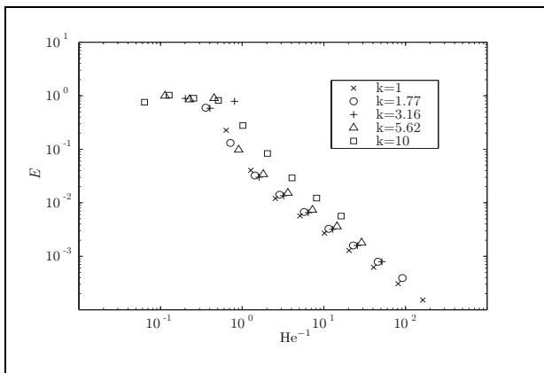
BILD 2. Mittlerer quadratischer Fehler E in Abhängigkeit von der inversen Helmholtzzahl für verschiedene Wellenzahlen k .
