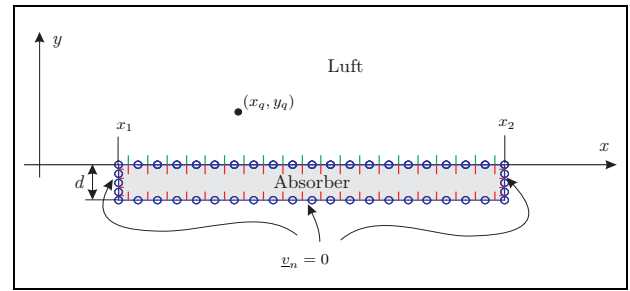
BILD 3. Geometrie: eine Zylinderquelle über einem Absorberstreifen
