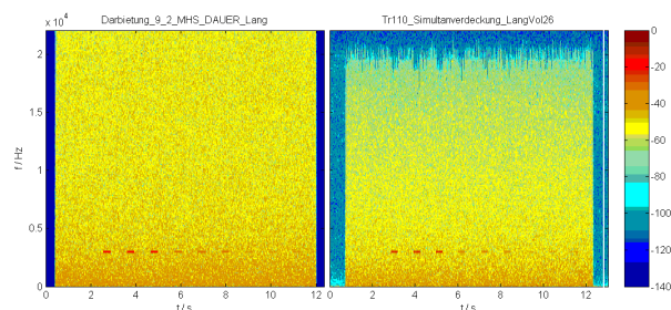
Abbildung 5: Campbell-Diagramm Simultanverdeckung mit 300 ms Impulsgruppen abnehmender Amplitude, links Originalsignal, rechts MD-Aufnahme
