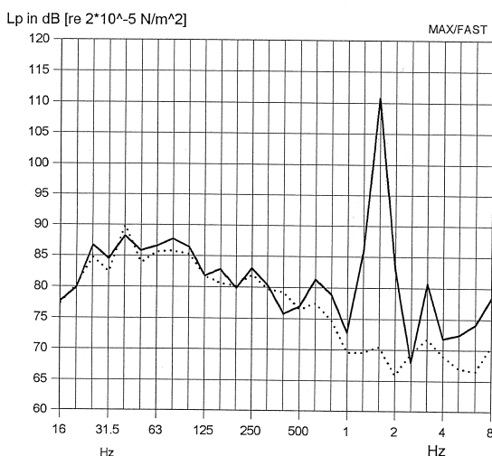
Bild 1: Straßenbahnpegel mit/ohne Quietschgeräusch
