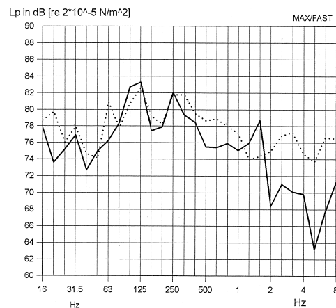
Bild 2: Straßenbahnpegel mit/ohne Zischelgeräusch
