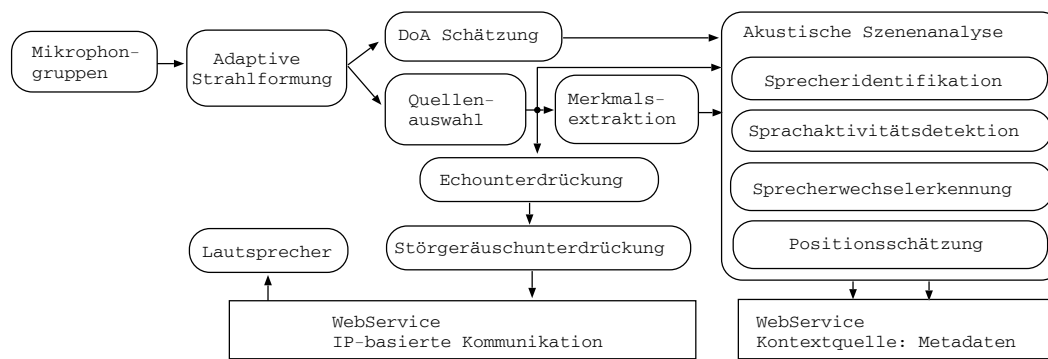
Abbildung 2: Akustische Szenenanalyse
