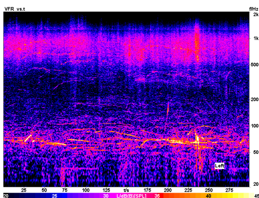
Abb. 1: Umweltgeräusch in größerer Entfernung zu einer Autobahn. VFR vs. time. (SPL in dB(B))
