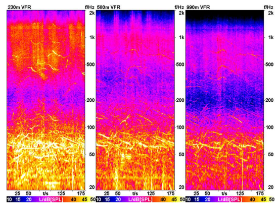
Abb. 2: Umweltgeräusch in unterschiedlichen Entfernungen (230m, 580m, 990m) zu einer Autobahn. VFR vs. time. (SPL in dB)
