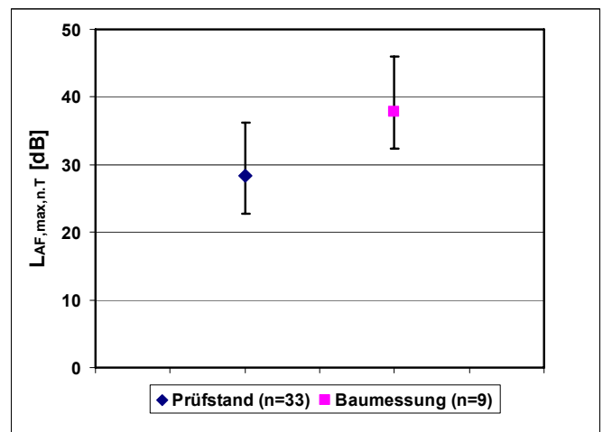
Bild 2: Vergleich von Prüfstands- und Baumessungen, WC, diagonale Messrichtung
