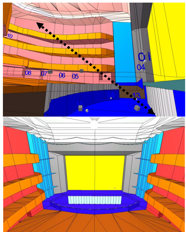
Abbildung 2: DOR, Simulationen Maßnahmen oben: seit 2007 mit neuen Diffusoren im OG unten: seit 2010 neu: Proszenium+Reflektoren
