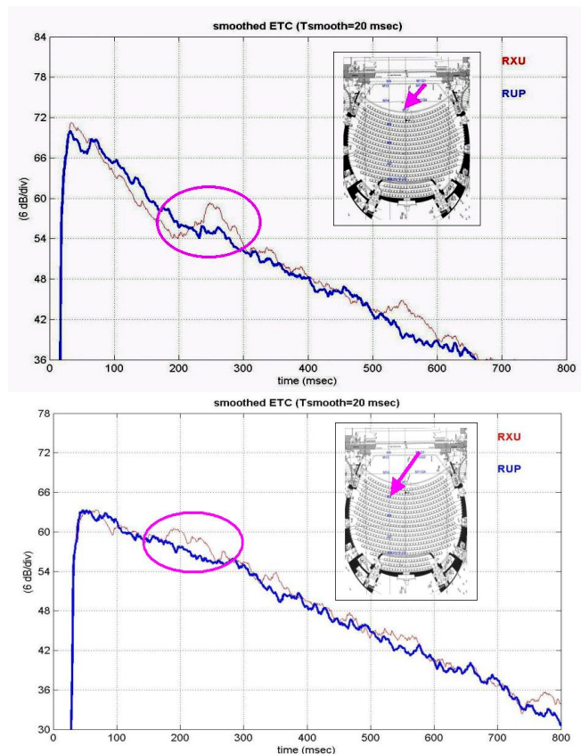
Abbildung 1: Echos und Effekt der Maßnahmen darauf: Vorher: rote Kurve, derzeit: blaue Kurve
