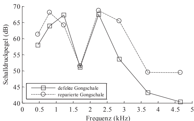
Abbildung 3: Maximalpegel der einzelnen Teiltöne der Gongschale vor (Quadrate) bzw. nach (Kreise) der Reparatur.
