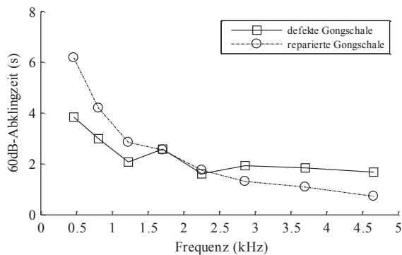
Abbildung 2: 60 dB-Abklingzeiten der einzelnen Teiltöne der Gongschale vor (Quadrate) bzw. nach (Kreise) der Reparatur.
