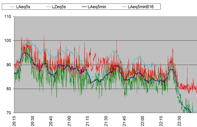
Abbildung 6: Pegelverlauf während des Spiels im Familien-Block als Kurzzeitmittelwert (5 s) unbewertet (rot) und A-bewertet (grün). In dunkelblau der Verlauf des 5 Minuten Mittelungspegels.
