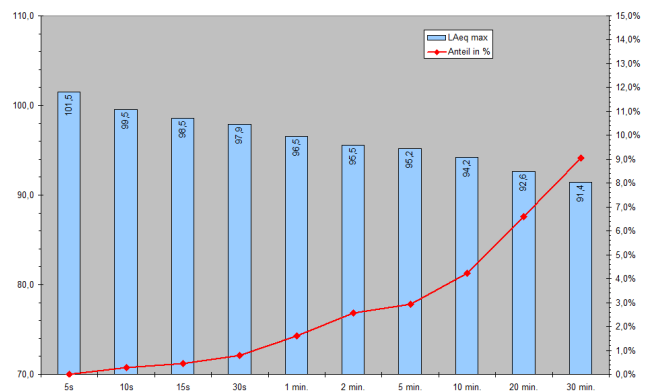
Abbildung 8: Siehe Abbildung 7 für Messwerte aus dem Familien-Block.
