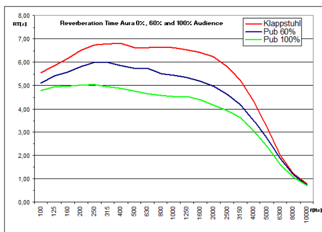
Abbildung 1: Berechnete Nachhallzeitverläufe für ein großes Sportstadion in Abhängigkeit von der Besetzung.
