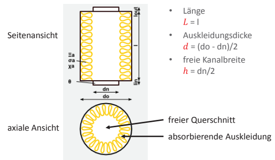
Abbildung 3: Schematische Darstellung eines Absorptionsschalldämpfers ohne Kulisse.
