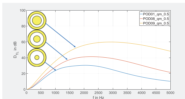
Abbildung 11: D_{TL} von Absorptionsschalldämpfern mit Kulisse entsprechend der Geometrien in Tabelle 3 mit Massenfluss von 0,5 kg/s.
