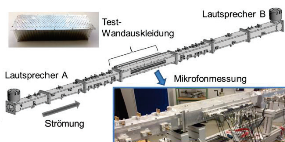
Abbildung 4: Strömungskanal und Messaufbau zur Impedanzbestimmung: Messung des Schalldruckverlaufs an der harten Wand gegenüber der Wandauskleidung zur Auswertung.
