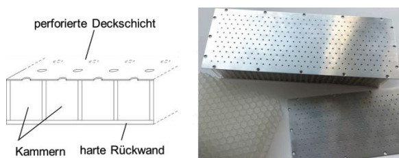
Abbildung 1: Aufbau einer resonatorartigen, schalldämpfenden Wandauskleidung (links) und Beispiel für eine Test-Auskleidung bestehend aus einer runden Zellstruktur und einem dünnen Lochblech (rechts).
