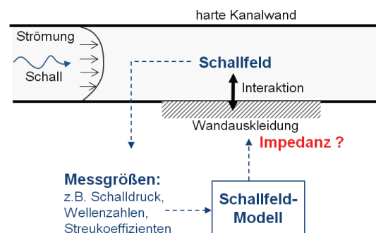
Abbildung 2: Prinzip der Impedanzbestimmung für eine akustische Wandauskleidung in einem Strömungskanal.
