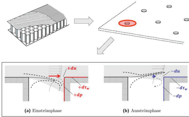
Abbildung 5: 2D-Ansicht einer einzelnen Öffnung des Lochblechs mit stationärer Überströmung für zwei Phasen der Durchströmung der Öffnung. Eingezeichnet ist die an der Vorderkante ablösende Wand-Stromlinie und die an der Hinterkante infolge der Durchströmung wirkende Änderung der Längsgeschwindigkeit du , des Drucks dp und der Wandschubspannung d\tau_w .
